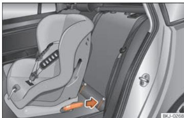
SL 39 Stražnja sjedala: ugradnja dječje sjedalice s ISOFIX sustavom.
