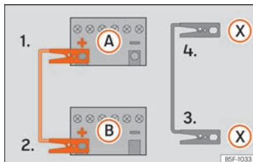
Sl. 155 Shema priključivanja za vozila sa start-stop sustavom.
