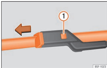
SL. 152 Zamjena prednjih metlica brisača.
