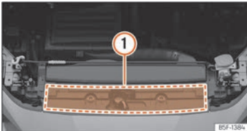
Sl. 177 U prostoru motora: položaj naljepnice sa specifikacijama motornog ulja
