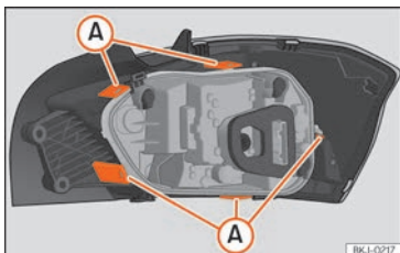
Sl. 164 Pričvrstne omče na poledini stražnjeg svjetla.
