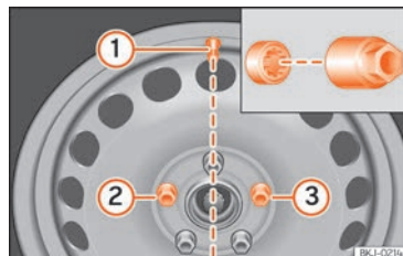
Sl. 190 Zamjena kotača: ventil gume ① i mjesto ugradnje vijka kotača sa zaštitom od krađe ② ili ③.
