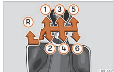
Sl. 89 Shema mijenjanja stupnjeva prijenosa kod ručnog mjenjača s 5 odn. 6 stupnjeva prijenosa
