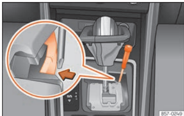
Sl. 93 Ručica automatskog mjenjača: deblokiranje iz položaja parkiranja
