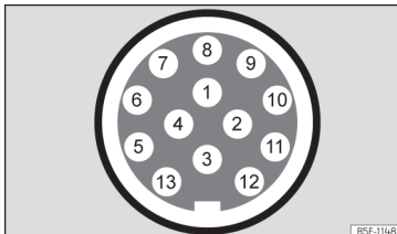
Sl. 143 Shematski prikaz: raspored zatika utičnih spojeva za struju prikolice.
